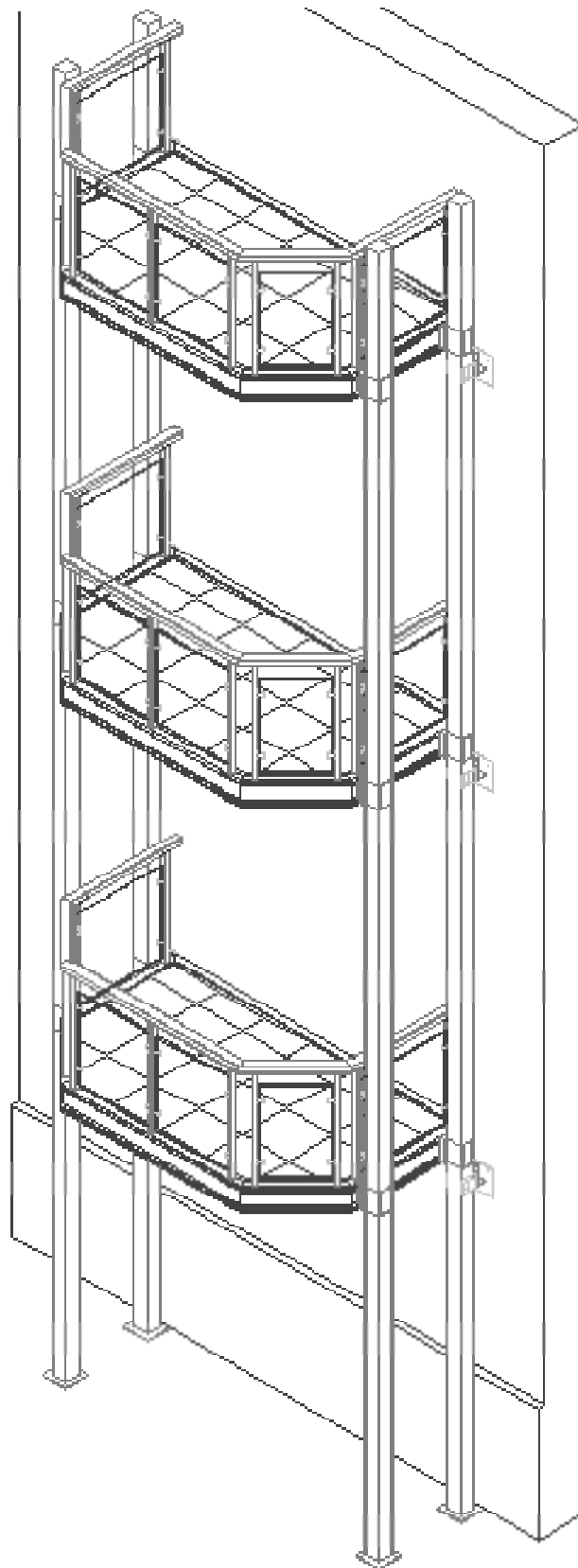
ANBAUBALKON LEICHTBAUVARIANTE GELÄNDER LM-E, VARIANTE PFOSTEN SICHTBAR.
