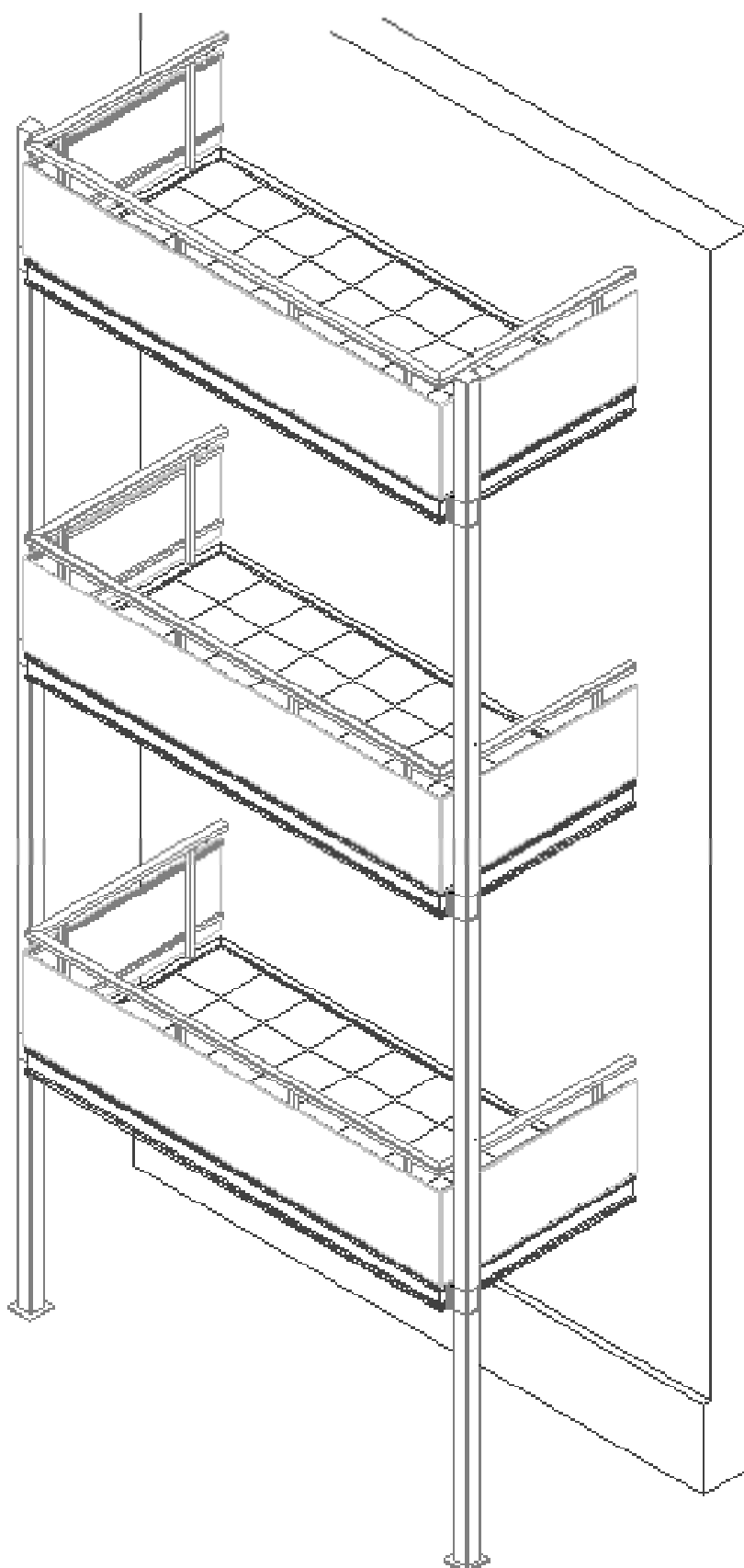
ANBAUBALKON LEICHTBAUVARIANTE GELÄNDER LM-E, VARIANTE PFOSTEN VERDECKT.
