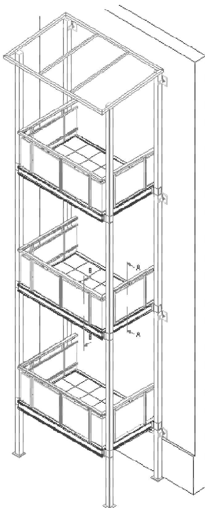
ANBAUBALKON LEICHTBAUVARIANTE GELÄNDER LM-E, VARIANTE PFOSTEN SICHTBAR.
