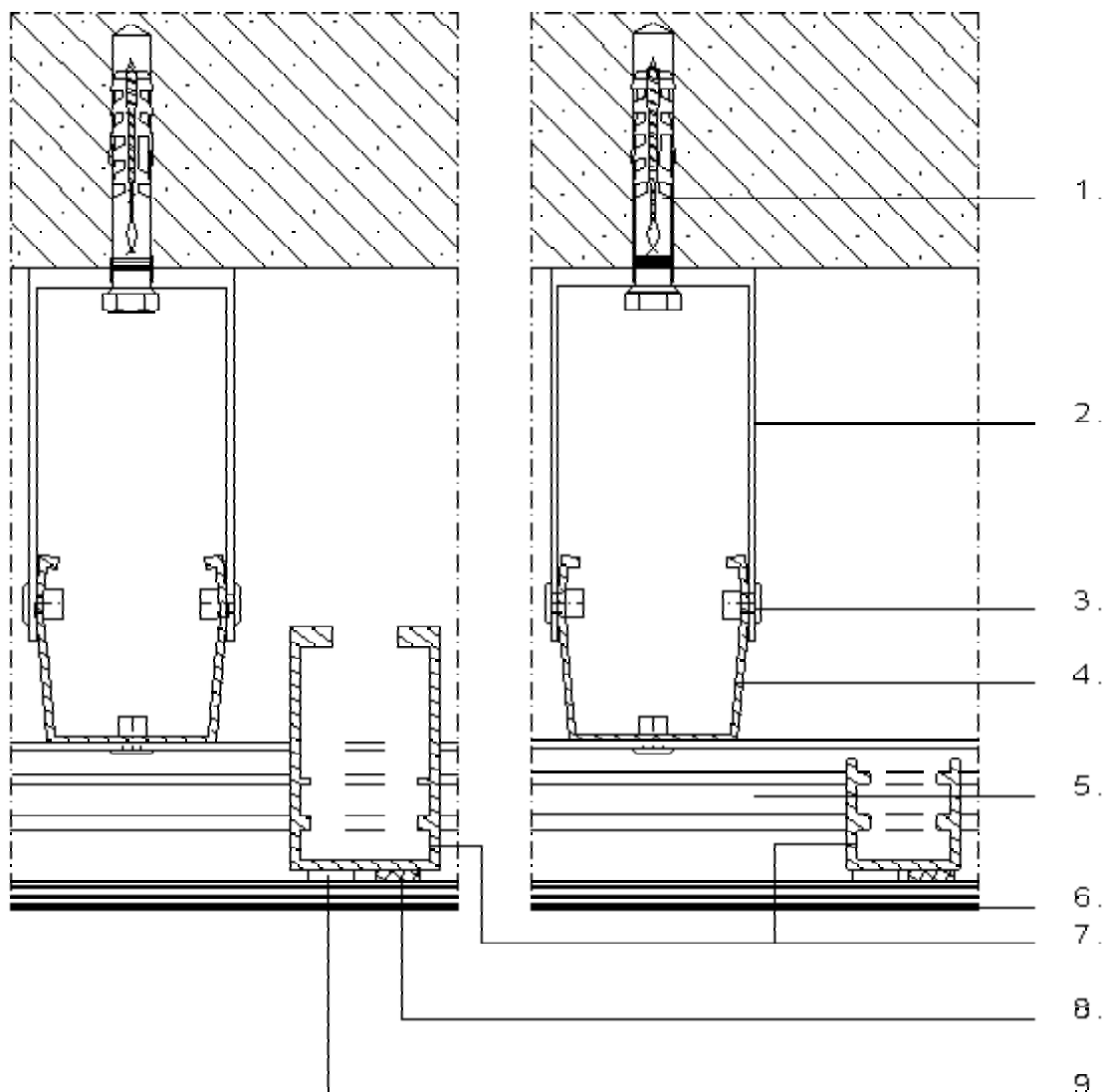
Plattentragprofil U2
